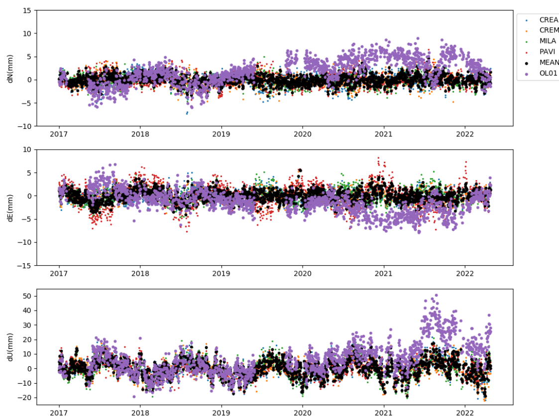
Figura 15 - Residui delle serie temporali NORTH, EAST, UP delle stazioni GNSS considerate nell'analisi. In colore sullo sfondo, i residui delle stazioni di riferimento: CREA, punti azzurri; CREM, punti arancioni; PAVI, punti rossi; MILA e MIL2, punti verdi (MILA e MIL2 sono state unite assieme per ricoprire l'intero arco temporale 2017-2022). In viola, in primo piano, la stazione OL01 a cui è stato tolto il trend delle altre stazioni. In nero la media dei residui delle stazioni di riferimento. Per "agganciare" le serie temporali ed evidenziare, graficamente, l'anomalia di OL01 abbiamo considerato come zero la media di OL01 calcolata dall'inizio fino a giugno 2019 (in corrispondenza dell'interruzione di dati).
