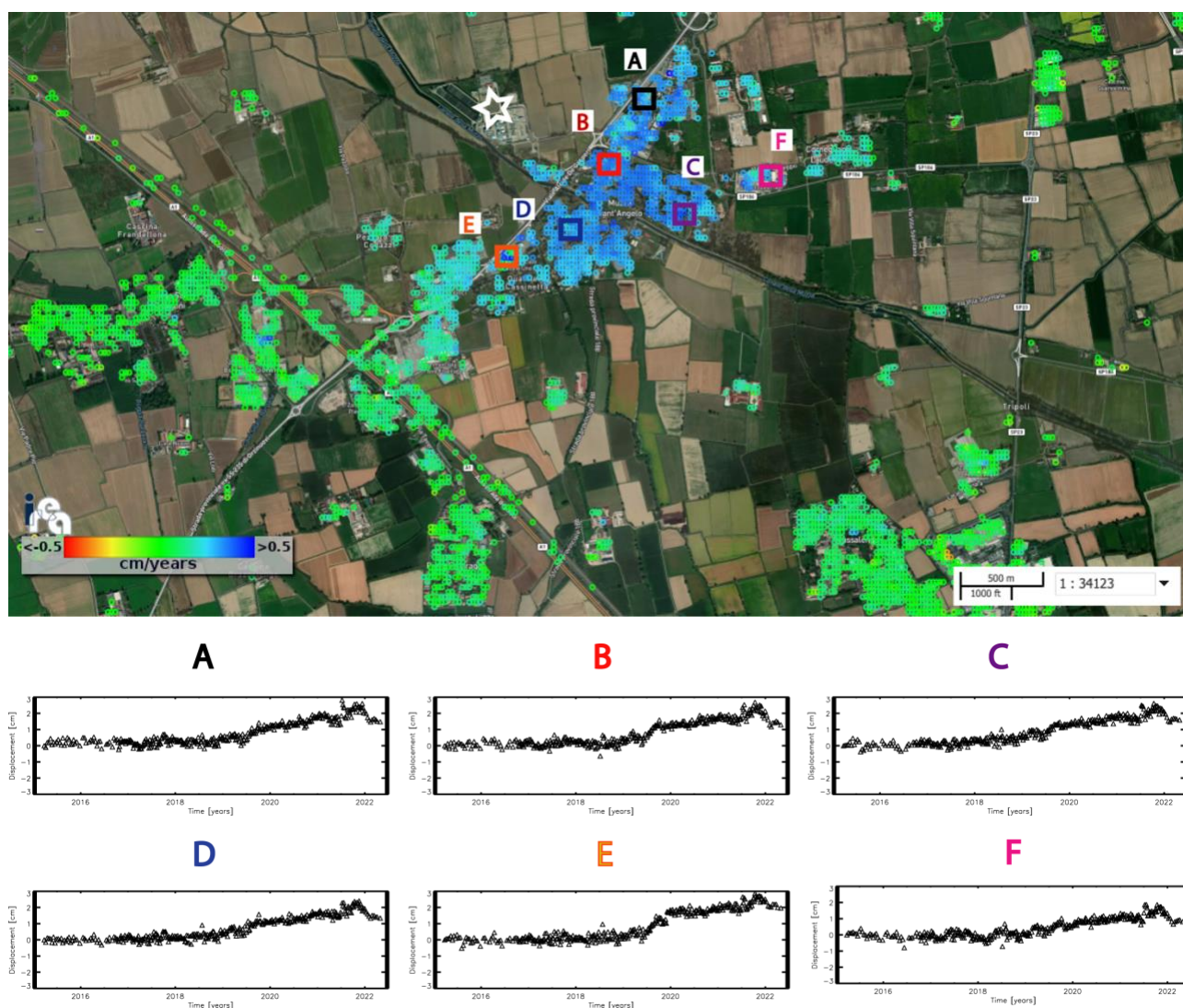
Figura 27 - Zoom della mappa della componente verticale della velocità di deformazione sull'area di Cornegliano Laudense situata in prossimità del sito di stoccaggio (la stellina bianca corrisponde al Cluster A). Sono inoltre mostrate le serie temporali della componente verticale dello spostamento superficiale di tutti i pixel evidenziati tramite i rettangoli colorati A-F sulla mappa di deformazione.
