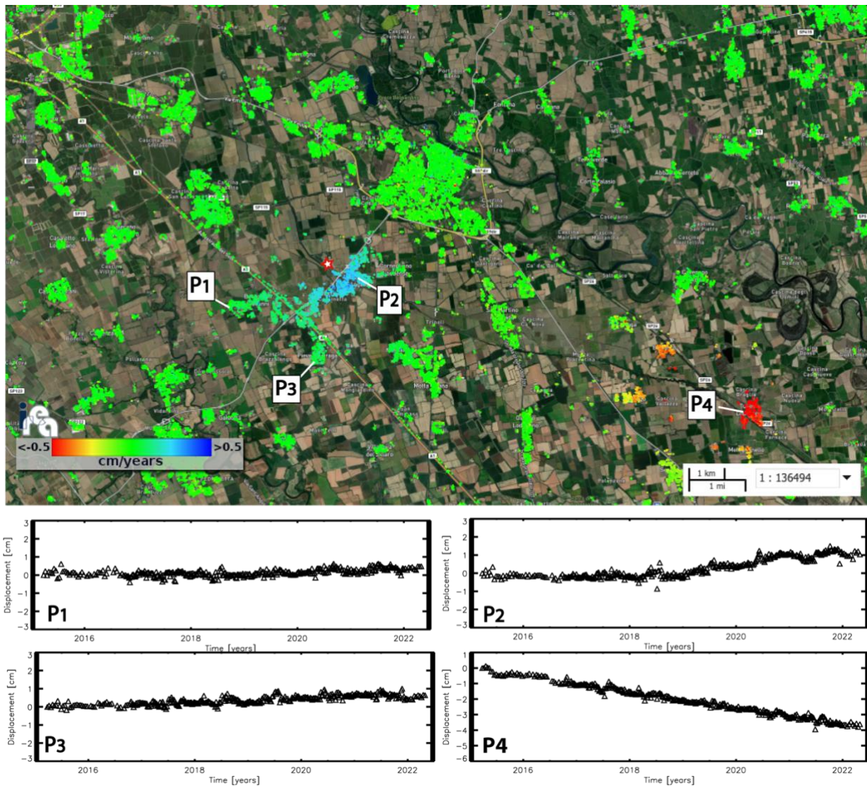
Figura 22 - Zoom della mappa di velocità media di deformazione di Figura 21 in corrispondenza dell'area identificata dal rettangolo bianco, incentrata sull'area che comprende i comuni di Cornegliano Laudense e di Turano Lodigiano. La stellina con contorno rosso indica la posizione dell'impianto di stoccaggio (Cluster A). I grafici riportano l'andamento temporale dello spostamento superficiale in LOS per tre punti localizzati nei pressi di Cornegliano Laudense (P1, P2 e P3) e un punto localizzato nell'area di Turano Lodigiano (P4). L'immagine si riferisce alla elaborazione dei dati S-1 acquisiti da orbite ascendenti nel periodo marzo 2015 - aprile 2022.
