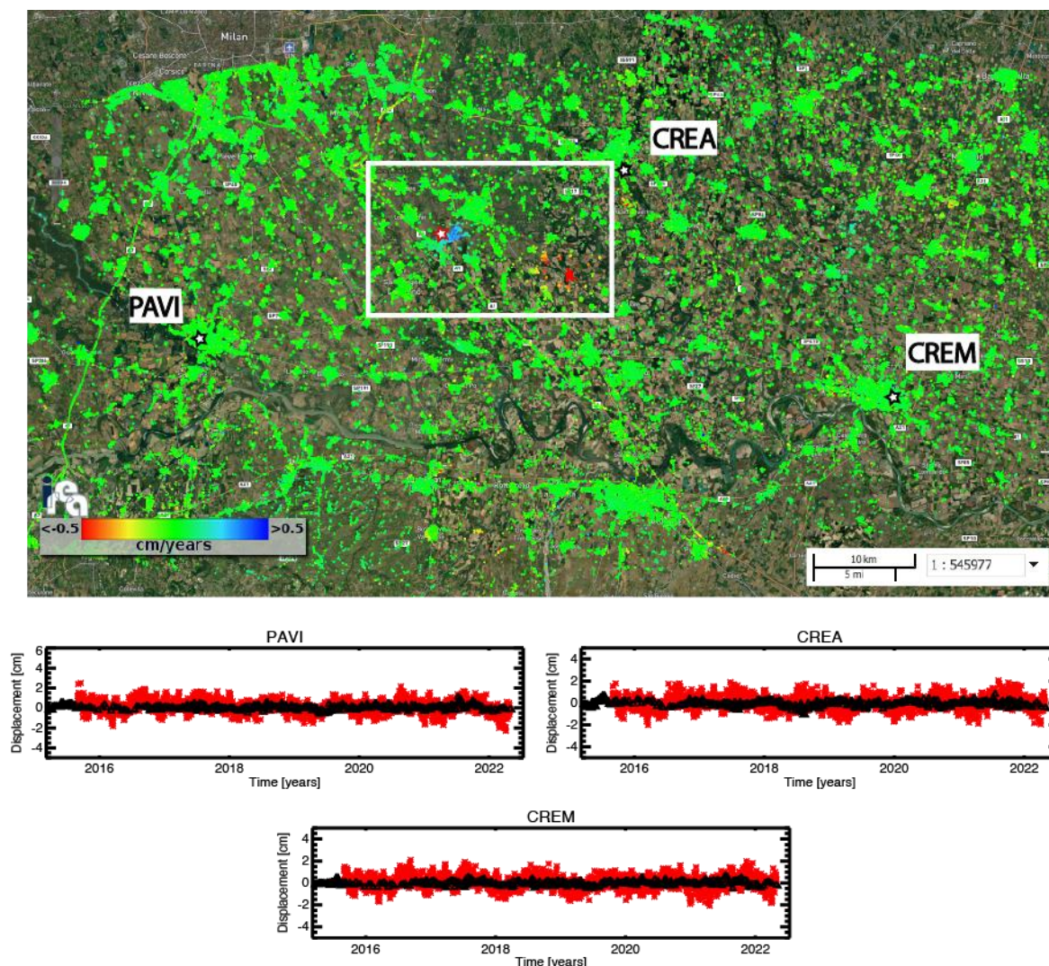
Figura 23 - Mappa della componente verticale della velocità di deformazione, geocodificata ed espressa in cm/anno, sovrapposta ad un'immagine ottica dell'area di interesse. La stellina rossa nel riquadro bianco indica il sito dell'impianto di stoccaggio. Si riportano, inoltre, in corrispondenza delle 3 stazioni GPS identificate sulla mappa tramite stelline nere, i grafici dei confronti tra la componente verticale delle serie storiche di deformazione GPS (asterischi rossi) e quella ottenute tramite i dati DInSAR (triangoli neri).
