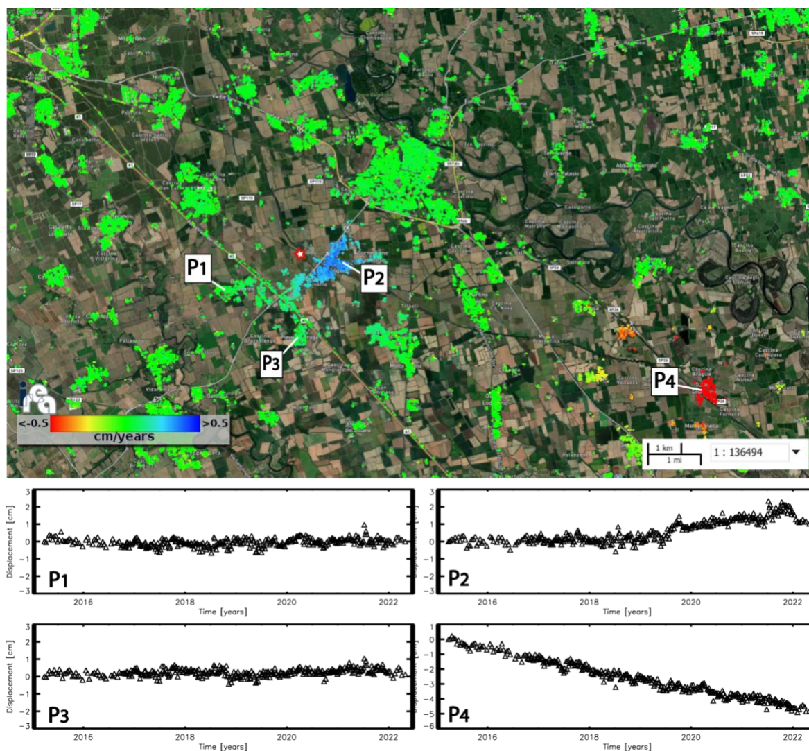
Figura 25 - Zoom della mappa della componente verticale della velocità media di deformazione di Figura 23 in corrispondenza del riquadro bianco, incentrato sull'area che comprende i comuni di Cornegliano Laudense e di Turano Lodigiano. La stellina rossa indica la posizione dell'impianto di stoccaggio (Cluster A). I grafici riportano l'andamento temporale della componente verticale dello spostamento superficiale per tre punti localizzati in prossimità di Cornegliano Laudense (P1, P2 e P3) e un punto localizzato nell'area di Turano Lodigiano (P4).
