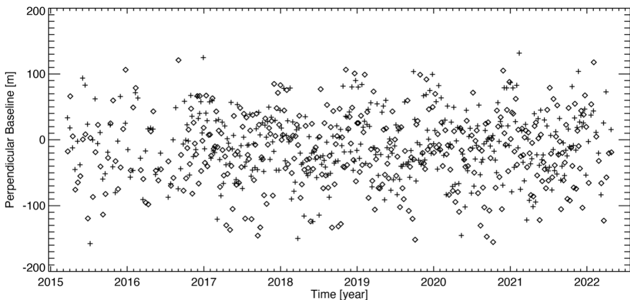
Figura 16 - Distribuzione nel piano tempo/baseline-perpendicolare dei dati SAR S-1 acquisiti sull'area di interesse. Ogni crocetta rappresenta un'immagine SAR acquisita da orbite discendenti, ogni rombo un'immagine SAR ottenuta da orbite ascendenti.
