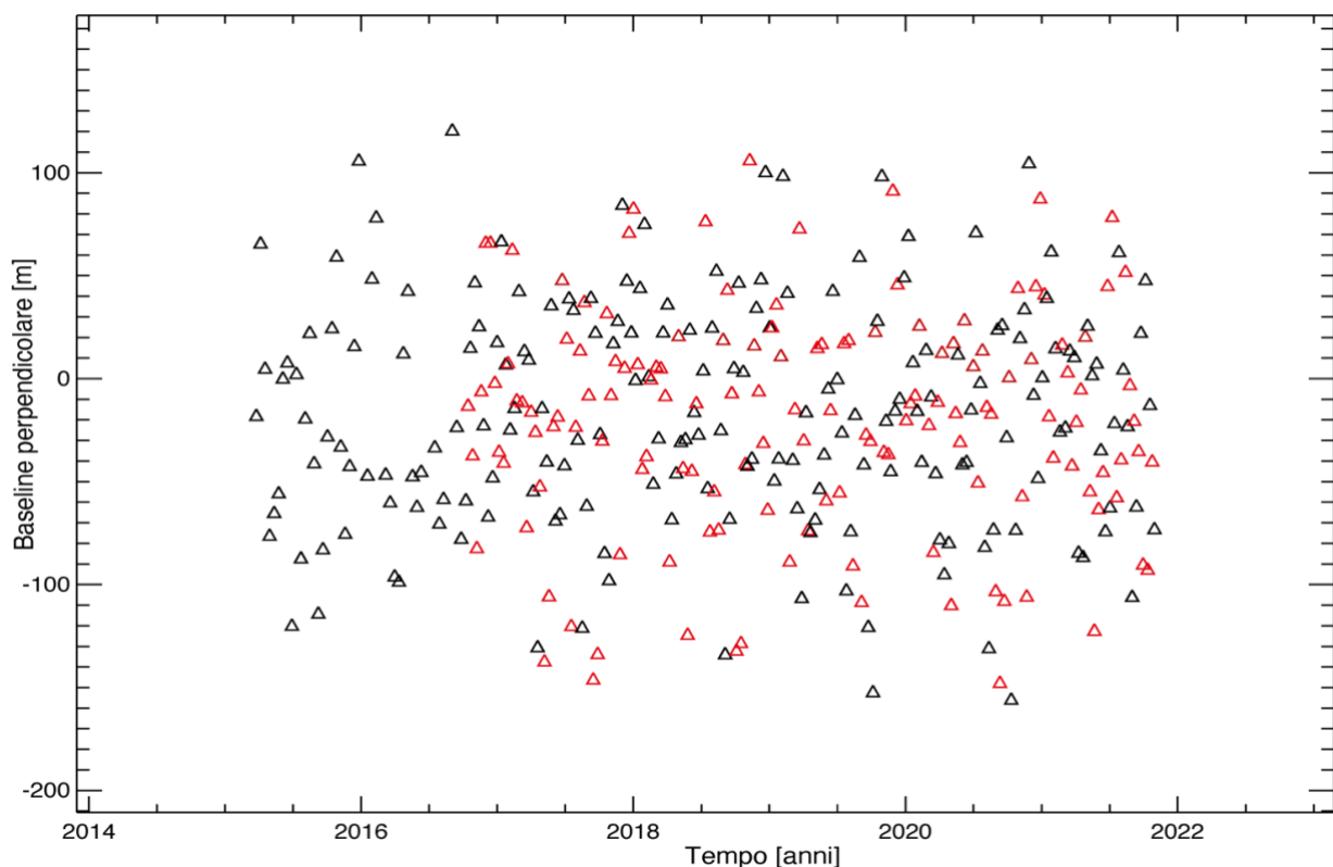
Figura 20 - Distribuzione nel piano tempo/baseline perpendicolare dei dati SAR S-1 acquisiti da orbite ascendenti sull'area di interesse. I triangoli neri e rossi rappresentano rispettivamente i dati S-1A e S-1B.
