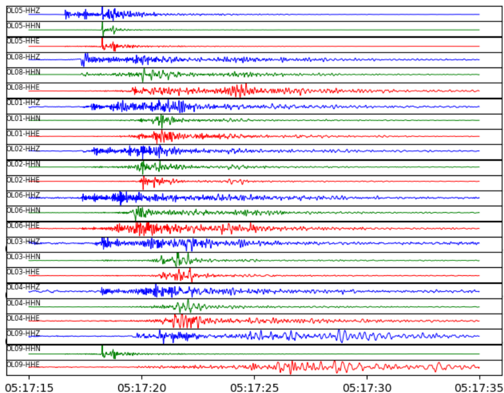
Figura 6 - Forme d'onda registrate per l'evento ML2.2 del 22/11/2021 ore 05:17:17 avvenuto nel Dominio Esterno. Sono raffigurate tre componenti per ogni stazione (la componente verticale è in colore blu). Le tracce sono quelle registrate dai sismometri posti in pozzo dalle seguenti stazioni, ordinate dall'alto verso il basso in base alla distanza dall'evento: OL05, OL08, OL01, OL02, OL06, OL03, OL04 e OL09.
