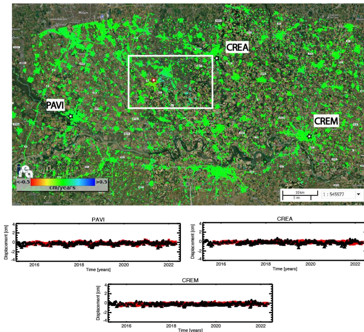
Figura 24 - Mappa della componente Est-Ovest della velocità di deformazione, geocodificata ed espressa in cm/anno, sovrapposta ad un'immagine ottica dell'area di interesse. La stellina rossa nel riquadro bianco indica il sito dell'impianto di stoccaggio. Si riportano, inoltre, in corrispondenza delle 3 stazioni GPS identificate sulla mappa tramite stelline nere, i grafici dei confronti tra le serie storiche di deformazione GPS in direzione Est-Ovest (asterischi rossi) e quelle ottenute tramite i dati DInSAR (triangoli neri).
