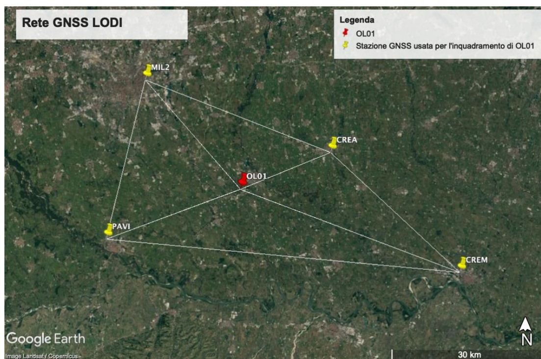
Figura 8 - Localizzazione delle stazioni GNSS utilizzate per l'inquadramento di OL01. Queste stazioni sono CREA (Crema), CREM (Cremona), MIL2 (Milano), PAVI (Pavia). La posizione della stazione MILA, rimasta attiva fino al 8/2/2019, è indistinguibile da quella di MIL2 in questo grafico.
