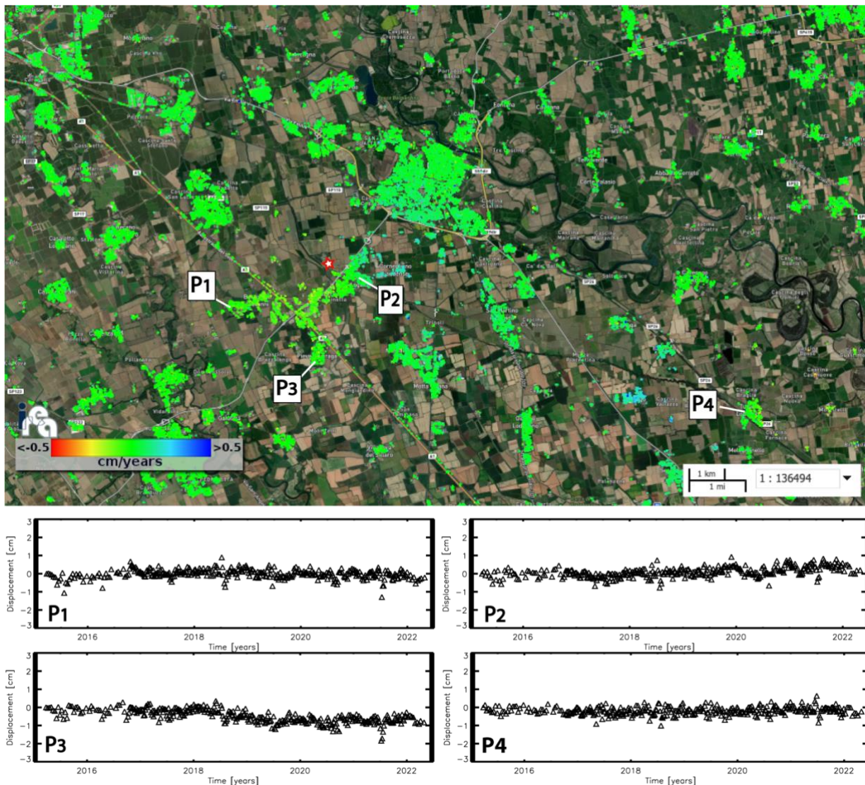
Figura 26 - Zoom della mappa della componente Est-Ovest della velocità media di deformazione Figura 24 in corrispondenza del riquadro bianco, incentrato sull'area che comprende i comuni di Cornegliano Laudense e di Turano Lodigiano. La stellina rossa indica la posizione dell'impianto di stoccaggio (Cluster A). I grafici riportano l'andamento temporale della componente Est-Ovest dello spostamento superficiale per tre punti localizzati in prossimità di Cornegliano Laudense (P1, P2 e P3) e un punto localizzato nell'area di Turano Lodigiano (P4).
