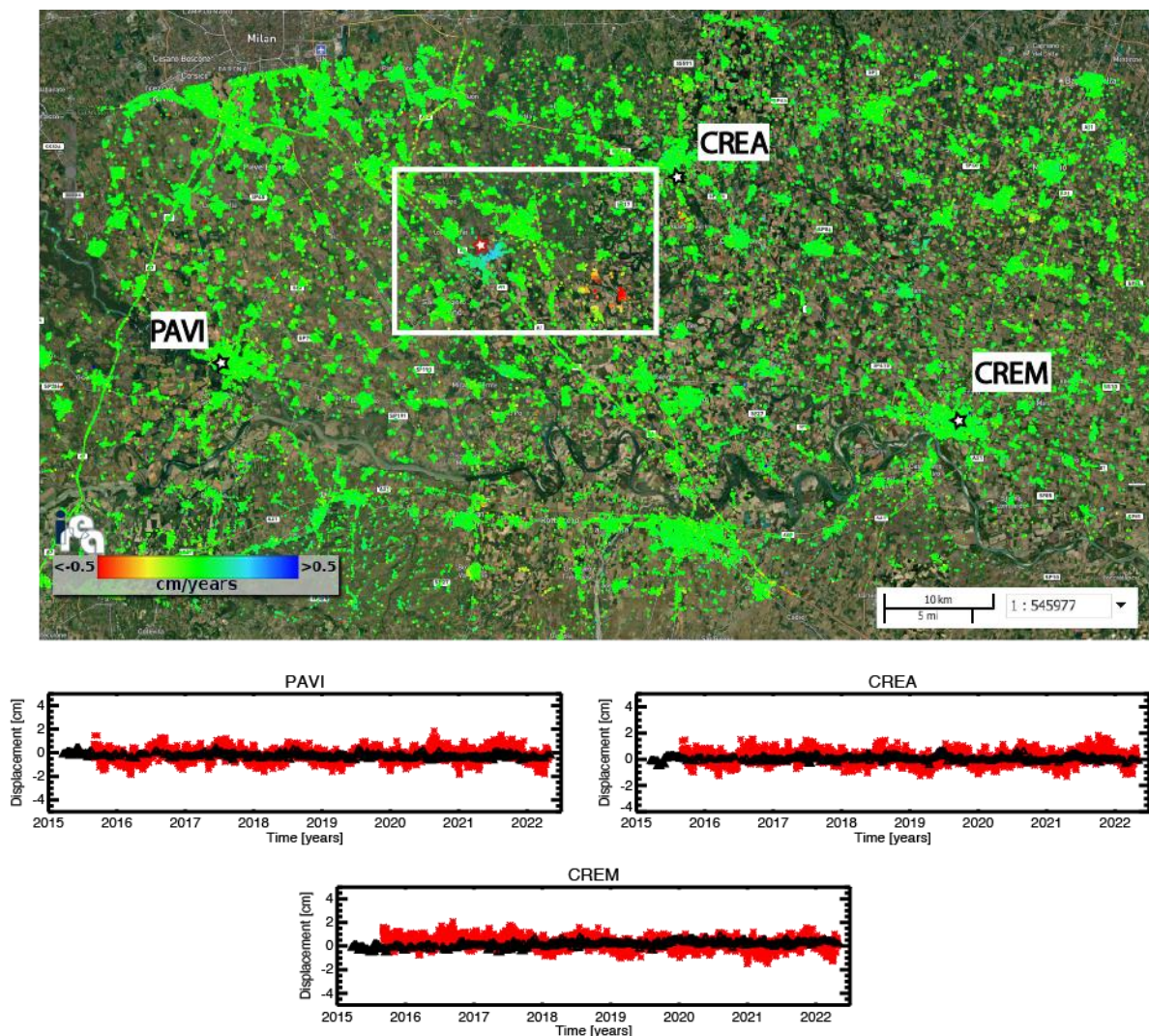
Figura 21 - Mappa di velocità di deformazione in LOS, geocodificata ed espressa in cm/anno, sovrapposta ad un'immagine ottica dell'area di interesse. L'immagine si riferisce alla elaborazione dei dati S-1 acquisiti da orbite ascendenti nel periodo marzo 2015 – aprile 2022. La stellina rossa nel riquadro bianco indica il sito dell'impianto di stoccaggio. Si riportano, inoltre, in corrispondenza delle 3 stazioni GPS identificate sulla mappa tramite stelline nere, i grafici dei confronti tra le serie storiche di deformazione GPS proiettate nella linea di vista del sensore radar (asterischi rossi) e quelle ottenute tramite i dati DInSAR (triangoli neri). Il rettangolo bianco fa riferimento alla zona analizzata in dettaglio in Figura 22 .
