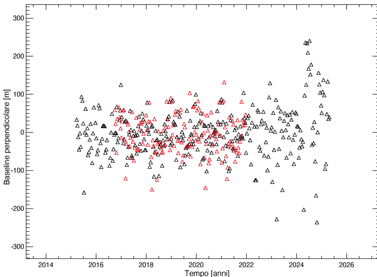
Figura 15 - Distribuzione nel piano tempo/baseline perpendicolare dei dati SAR S-1 acquisiti da orbite discendenti sull'area di interesse. I triangoli neri e rossi rappresentano rispettivamente i dati S-1A e S-1B. Si segnala l'assenza di acquisizioni S-1B a partire dal Dicembre 2021.
