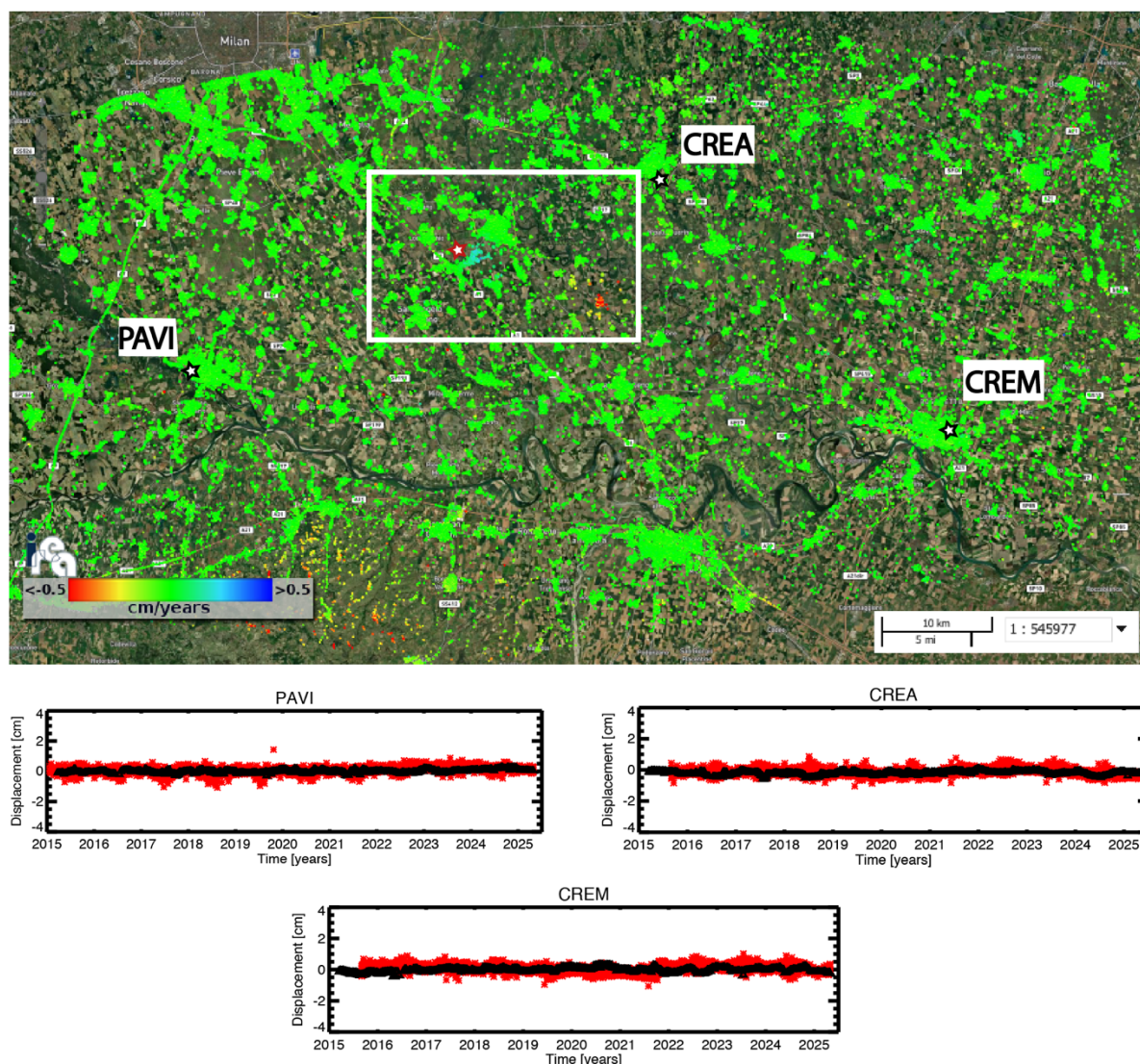
Figura 16 - Mappa di velocità di deformazione in LOS, geocodificata ed espressa in cm/anno, sovrapposta ad un'immagine ottica dell'area di interesse. L'immagine si riferisce alla elaborazione dei dati S-1 acquisiti da orbite discendenti nel periodo marzo 2015 - aprile 2025. La stellina rossa nel riquadro bianco indica il sito dell'impianto di stoccaggio. Si riportano, inoltre, in corrispondenza delle 3 stazioni GNSS identificate sulla mappa tramite stelline nere, i grafici dei confronti tra le serie temporali di deformazione GNSS proiettate nella linea di vista del sensore radar (asterischi rossi) e quelle ottenute tramite i dati DInSAR (triangoli neri). Il rettangolo bianco fa riferimento alla zona analizzata in dettaglio in Figura 17 .
