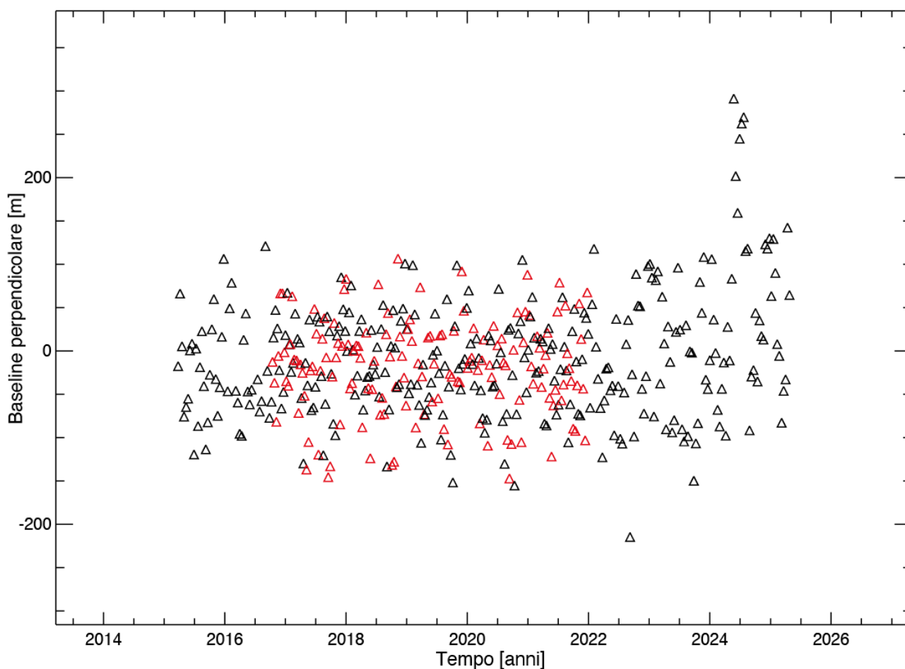
Figura 18 - Distribuzione nel piano tempo/baseline perpendicolare dei dati SAR S-1 acquisiti da orbite ascendenti sull'area di interesse. I triangoli neri e rossi rappresentano rispettivamente i dati S-1A e S-1B. Si segnala l'assenza di acquisizioni S-1B a partire dal Dicembre 2021.
