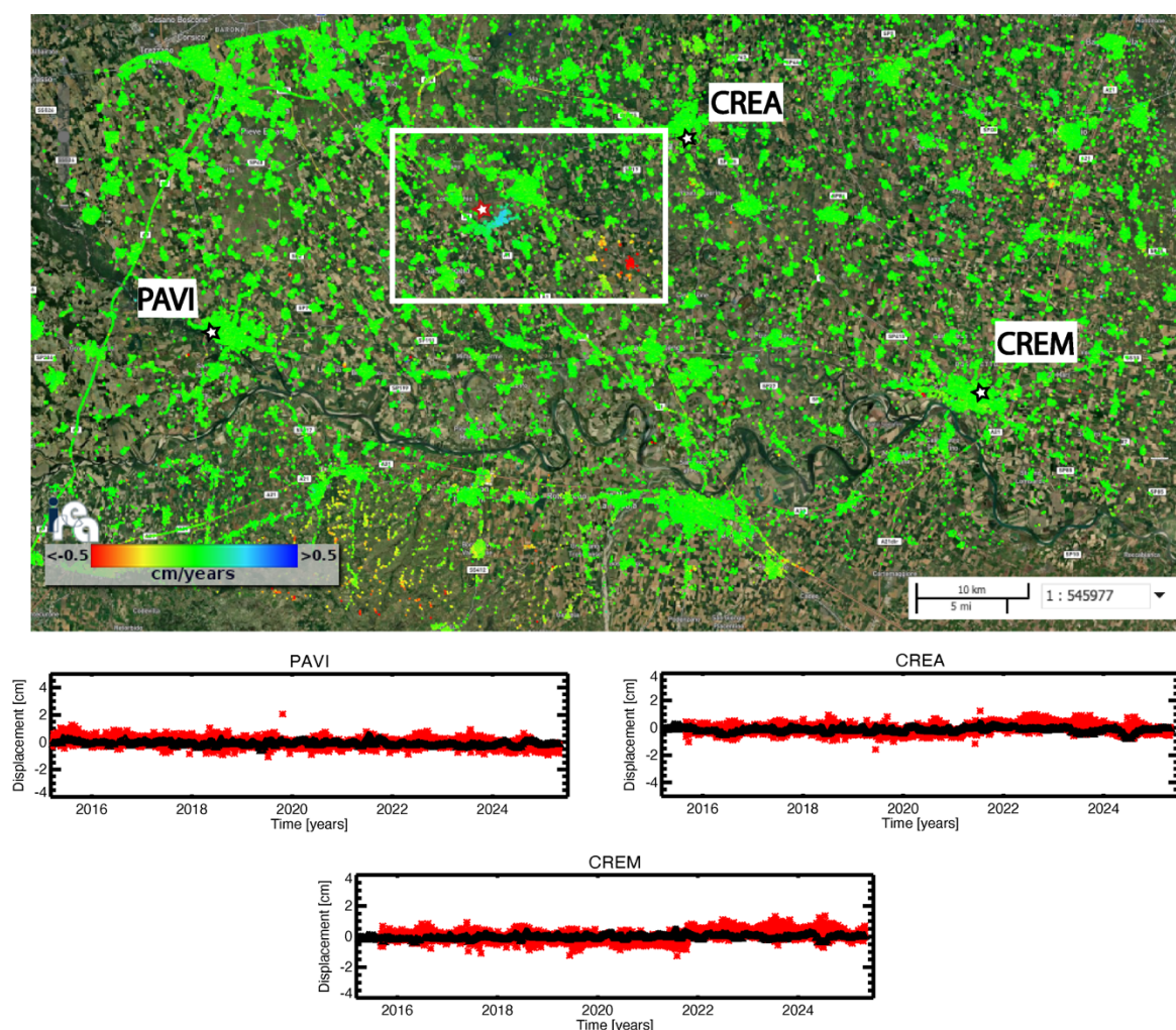
Figura 21 - Mappa della componente verticale della velocità di deformazione, geocodificata ed espressa in cm/anno, sovrapposta ad un'immagine ottica dell'area di interesse. La stellina rossa nel riquadro bianco indica il sito dell'impianto di stoccaggio. Si riportano, inoltre, in corrispondenza delle 3 stazioni GNSS identificate sulla mappa tramite stelline nere, i grafici dei confronti tra la componente verticale delle serie storiche di deformazione GPS (asterischi rossi) e quella ottenute tramite i dati DInSAR (triangoli neri). Il rettangolo bianco fa riferimento alla zona analizzata in dettaglio in Figura 23 .
