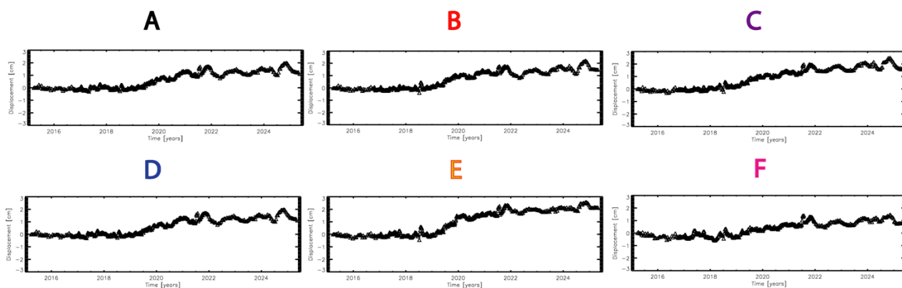
Figura 25 - Zoom della mappa della componente verticale della velocità di deformazione sull'area di Cornegliano Laudense situata in prossimità del sito di stoccaggio (la stellina bianca corrisponde al Cluster A). Sono inoltre mostrate le serie temporali della componente verticale dello spostamento superficiale di tutti i pixel evidenziati tramite i rettangoli colorati A-F sulla mappa di deformazione.
