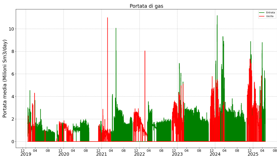
Figura 5 – (a) Pressione media misurata al collettore dei pozzi durante le attività dell'impianto del sito di Cornegliano Laudense. (b) Portata di gas (unità in milioni di metri cubi standard al giorno) durante le attività dell'impianto. In verde e rosso sono rappresentati rispettivamente i valori in entrata e uscita. (c) Volume complessivo del gas contenuto nel serbatoio naturale durante le attività dell'impianto, normalizzato al valore di volume massimo. I valori assoluti del volume sono mascherati di proposito in quanto rappresentano un dato commerciale sensibile e riservato. Continua alla pagina successiva.
