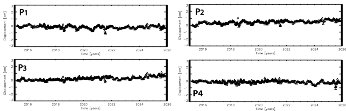
Figura 25 - Zoom della mappa della componente Est-Ovest della velocità media di deformazione Figura 24 in corrispondenza del riquadro bianco, incentrato sull'area che comprende i comuni di Cornegliano Laudense e di Turano Lodigiano. La stellina rossa indica la posizione dell'impianto di stoccaggio (Cluster A). I grafici riportano l'andamento temporale della componente Est-Ovest dello spostamento superficiale per tre punti localizzati in prossimità di Cornegliano Laudense (P1, P2 e P3) e un punto localizzato nell'area di Turano Lodigiano (P4).
