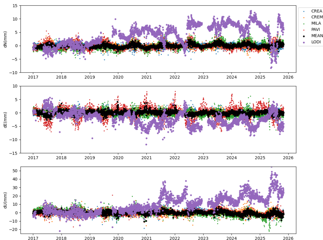
Figura 14 - Residui delle serie temporali Nord-Sud ( dN ), Est-Ovest ( dE ), Verticale ( dU ) delle stazioni GNSS considerate nell'analisi. In colore sullo sfondo, i residui delle stazioni di riferimento: CREA, punti azzurri; CREM, punti arancioni; PAVI, punti rossi; MILA, MIL2 e MIL3 punti verdi (MILA, MIL2 e MIL3 sono state unite insieme per ricoprire l'intero arco temporale 2017-2025). In viola, in primo piano, la stazione LODI a cui è stato tolto il trend delle altre stazioni. In nero la media dei residui delle stazioni di riferimento. Per evidenziare graficamente l'anomalia di LODI abbiamo considerato come zero la media di LODI calcolata sul periodo precedente all'inizio delle attività di stoccaggio.
