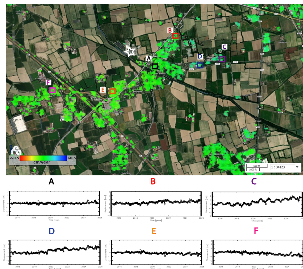
Figura 27 - Zoom della mappa della componente Est-Ovest della velocità di deformazione sull'area di Cornegliano Laudense situata in prossimità del sito di stoccaggio (la stellina bianca corrisponde al Cluster A). Sono inoltre mostrate le serie temporali della componente Est-Ovest dello spostamento superficiale di tutti i pixel evidenziati tramite i rettangoli colorati A-F sulla mappa di deformazione.
