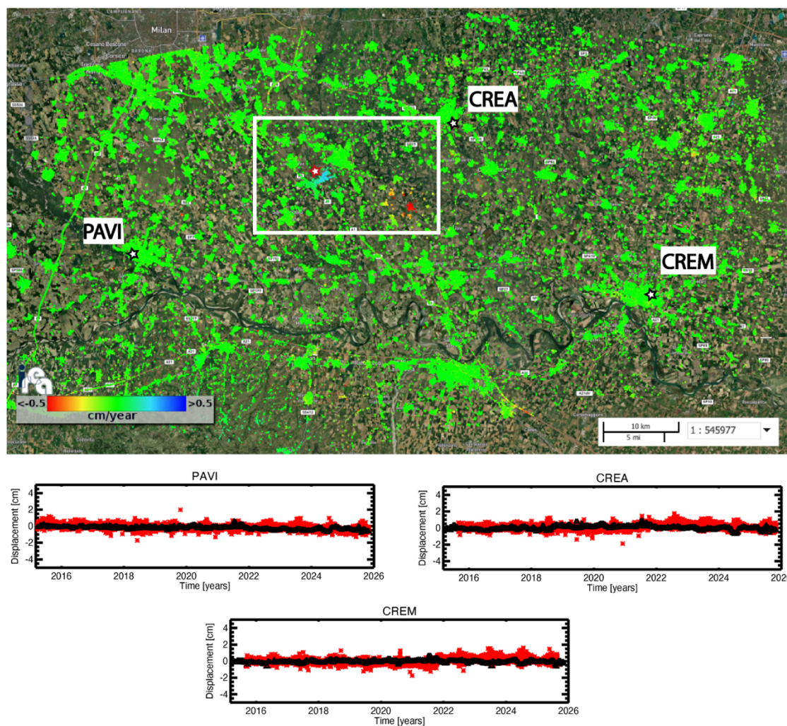
Figura 22 - Mappa della componente verticale della velocità di deformazione, geocodificata ed espressa in cm/anno, sovrapposta ad un'immagine ottica dell'area di interesse. La stellina rossa nel riquadro bianco indica il sito dell'impianto di stoccaggio. Si riportano, inoltre, in corrispondenza delle 3 stazioni GNSS identificate sulla mappa tramite stelline nere, i grafici dei confronti tra la componente verticale delle serie storiche di deformazione GNSS (asterischi rossi) e quella ottenute tramite i dati DInSAR (triangoli neri). Il rettangolo bianco fa riferimento alla zona analizzata in dettaglio in Figura 25.
