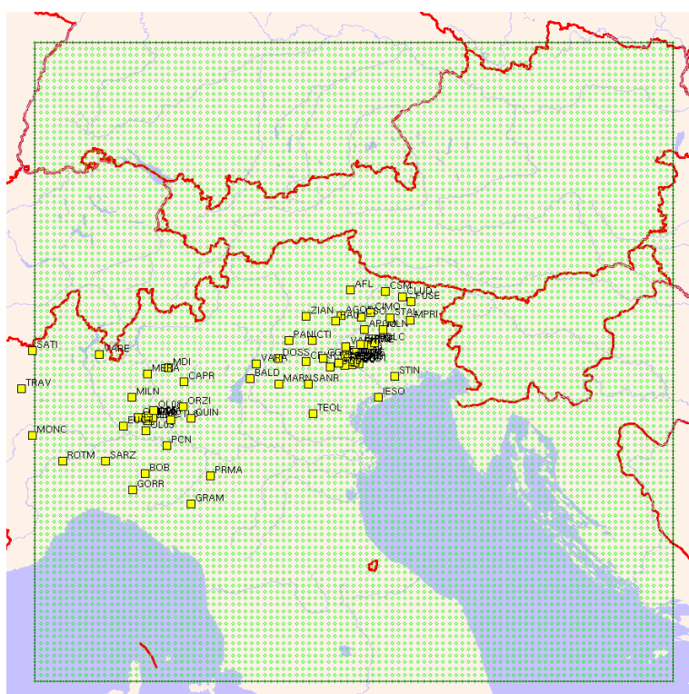
Figura 2. - Insieme delle stazioni sismometriche utilizzate dal sistema di monitoraggio sismico in cui è inserita la RMCL. Nell'area della Pianura Padana e nell'area Occidentale si riconoscono le stazioni di INGV e RSNI più vicine alla RMCL. Nell'area Orientale si distinguono invece le stazioni appartenenti alle reti gestite da OGS anche per conto delle Regioni Veneto e Friuli-Venezia Giulia, oltre alle stazioni della Provincia Autonoma di Trento. Il rettangolo punteggiato rappresenta l'area di riconoscimento dei terremoti regionali, indispensabile. Per evitare false identificazioni di eventi locali.
