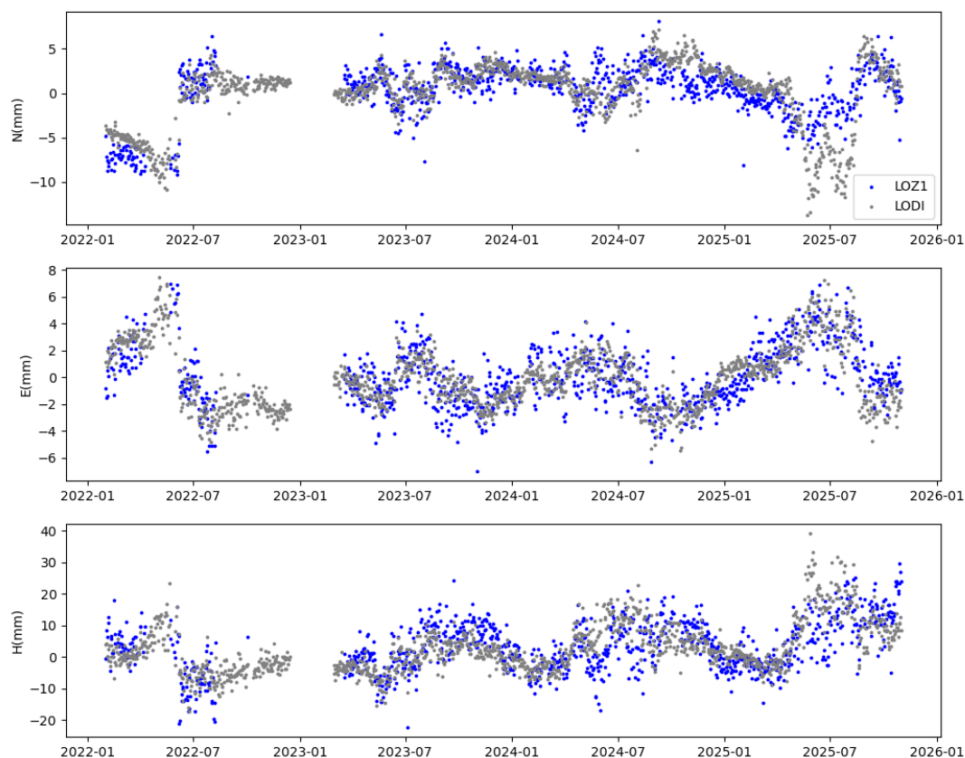
Figura E.2 - Serie temporali di LOZ1 (in blu) e di LODI (in grigio) dall'inizio di operatività di LOZ1 fino al giorno ultimo considerato nella presente relazione.
