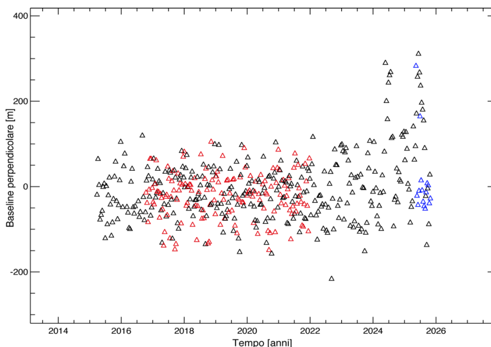
Figura 19 - Distribuzione nel piano tempo/baseline perpendicolare dei dati SAR S-1 acquisiti da orbite ascendenti sull'area di interesse. I triangoli neri, rossi e blu rappresentano rispettivamente i dati S-1A, S-1B e S-1C. Si segnala l'assenza di acquisizioni S-1B a partire da dicembre 2021 e la presenza di dati S-1C a partire da aprile 2025.
