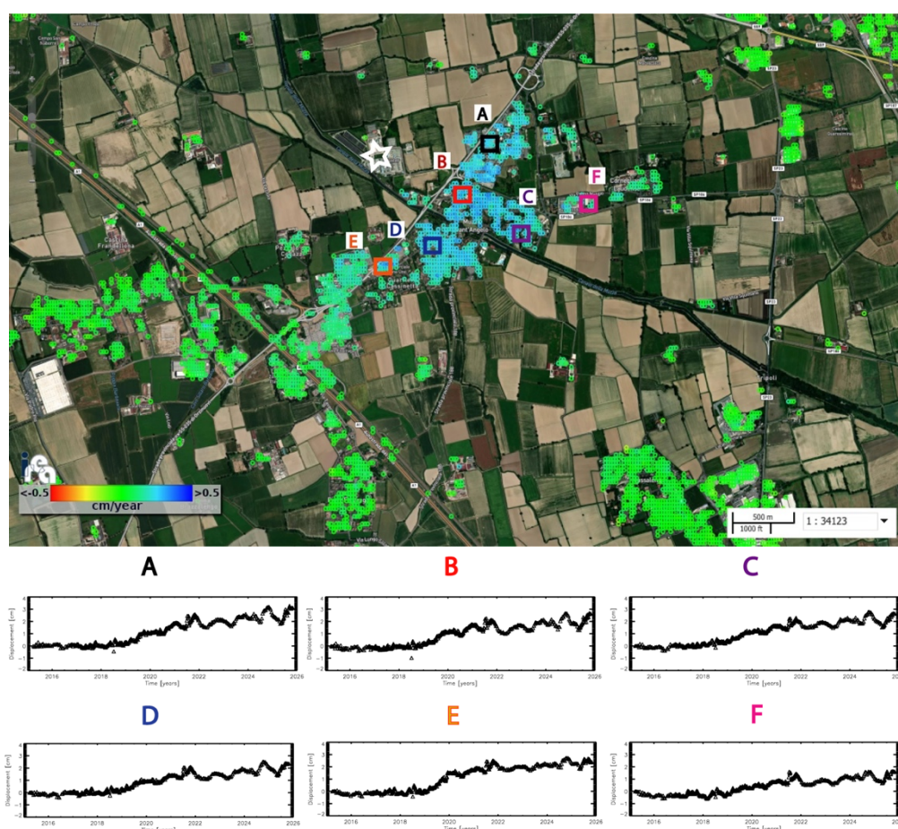
Figura 26 - Zoom della mappa della componente verticale della velocità di deformazione sull'area di Cornegliano Laudense situata in prossimità del sito di stoccaggio (la stellina bianca corrisponde al Cluster A). Sono inoltre mostrate le serie temporali della componente verticale dello spostamento superficiale di tutti i pixel evidenziati tramite i rettangoli colorati A-F sulla mappa di deformazione.
