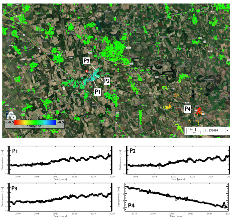
Figura 21 - Zoom della mappa di velocità media di deformazione di Figura 20 in corrispondenza dell'area identificata dal rettangolo bianco, incentrata sull'area che comprende i comuni di Cornegliano Laudense e di Turano Lodigiano. La stellina con contorno rosso indica la posizione dell'impianto di stoccaggio (Cluster A). I grafici riportano l'andamento temporale dello spostamento superficiale in LOS per tre punti localizzati nei
