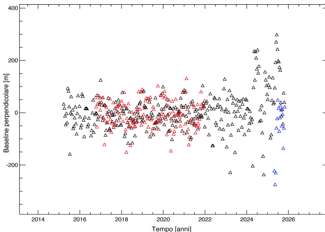
Figura 16 - Distribuzione nel piano tempo/baseline perpendicolare dei dati SAR S-1 acquisiti da orbite discendenti sull'area di interesse. I triangoli neri, rossi e blu rappresentano rispettivamente i dati S-1A, S-1B e S-1C. Si segnala l'assenza di acquisizioni S-1B a partire da dicembre 2021 e la presenza di dati S-1C a partire da aprile 2025.
