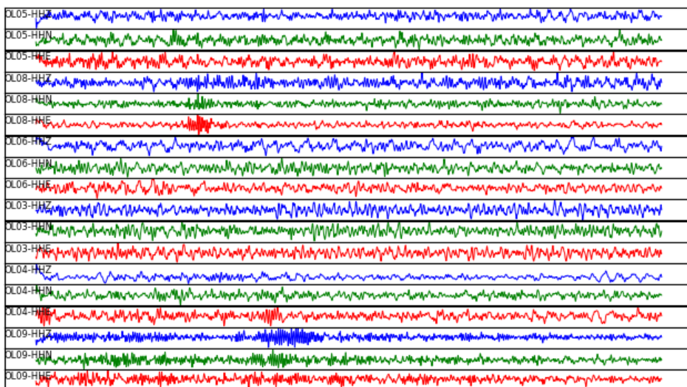
Figura 3 - Forme d'onda registrate per l'evento ML1.5 del 02/08/2025 ore 08:38:26 avvenuto nel Dominio Esteso. Sono raffigurate tre componenti per ogni stazione (la componente verticale è in colore blu, le due componenti orizzontali rispettivamente in rosso (E-O) e verde (N_S)). Le tracce sono quelle registrate sui sismometri posti in pozzo delle seguenti stazioni, ordinate dall'alto verso il basso in base alla distanza dall'evento: OL05, OL08, OL06, OL03, OL04, OL09.
