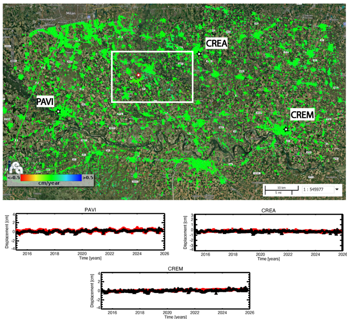
Figura 23 - Mappa della componente Est-Ovest della velocità di deformazione, geocodificata ed espressa in cm/anno, sovrapposta ad un'immagine ottica dell'area di interesse. La stellina rossa nel riquadro bianco indica il sito dell'impianto di stoccaggio. Si riportano, inoltre, in corrispondenza delle 3 stazioni GNSS identificate sulla mappa tramite stelline nere, i grafici dei confronti tra le serie storiche di deformazione GNSS in direzione Est-Ovest (asterischi rossi) e quelle ottenute tramite i dati DInSAR (triangoli neri). Il rettangolo bianco fa riferimento alla zona analizzata in dettaglio in Figura 25.
